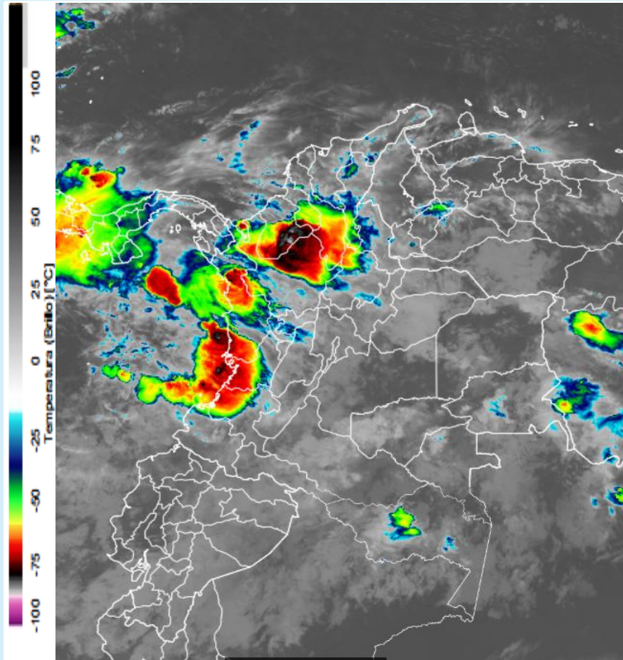
Imagen GOES 19 (East) Canal Infrarrojo 10 de julio de 2025 - Hora 23:30 HLC Fuente: IDEAM
