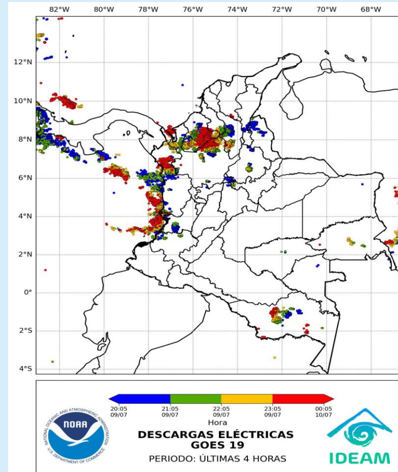
Descargas eléctricas 10 de julio de 2025 – Hora 23:30 HLC Fuente: IDEAM
