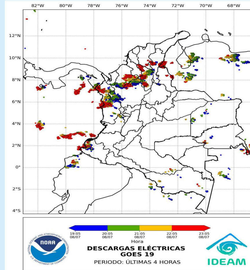
Descargas eléctricas 8 de julio de 2025 - Hora 23:05 HLC Fuente: IDEAM
