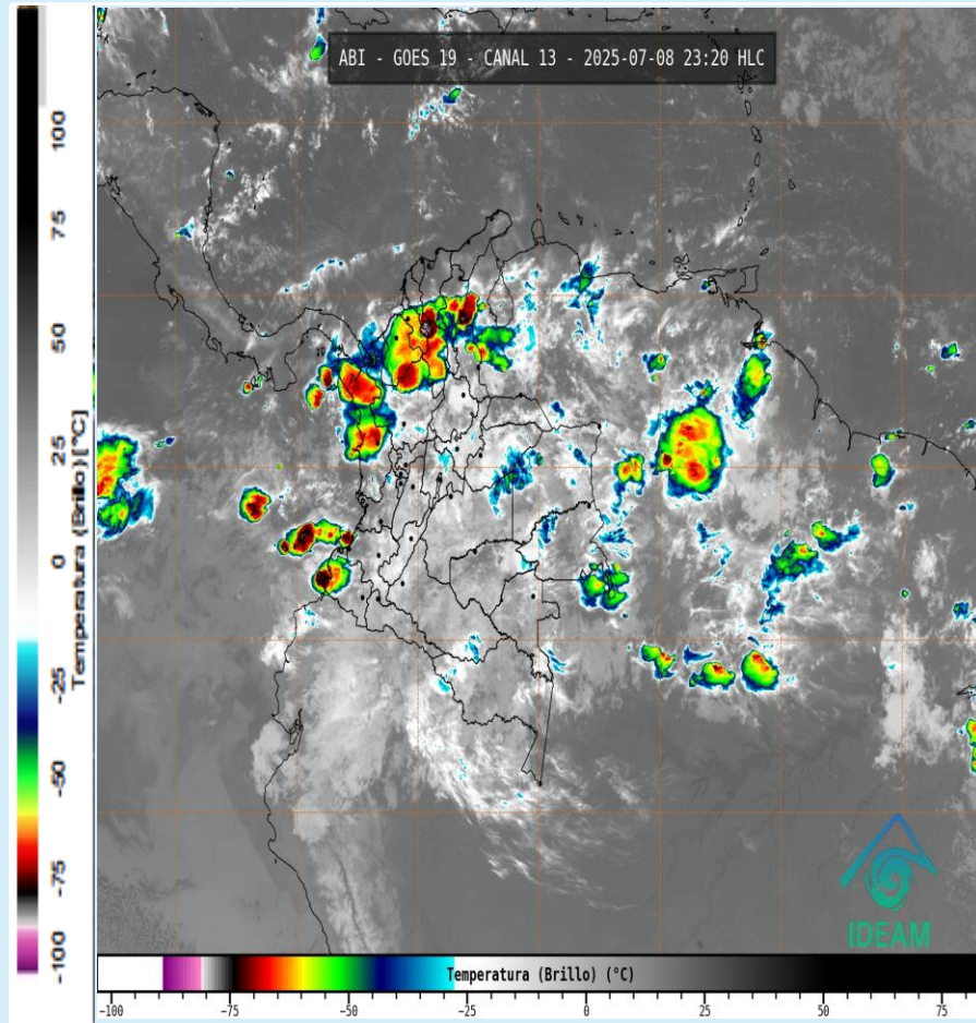
Imagen GOES 19 (East) Canal Infrarrojo 8 de julio de 2025 - Hora 23:20 HLC Fuente: IDEAM
