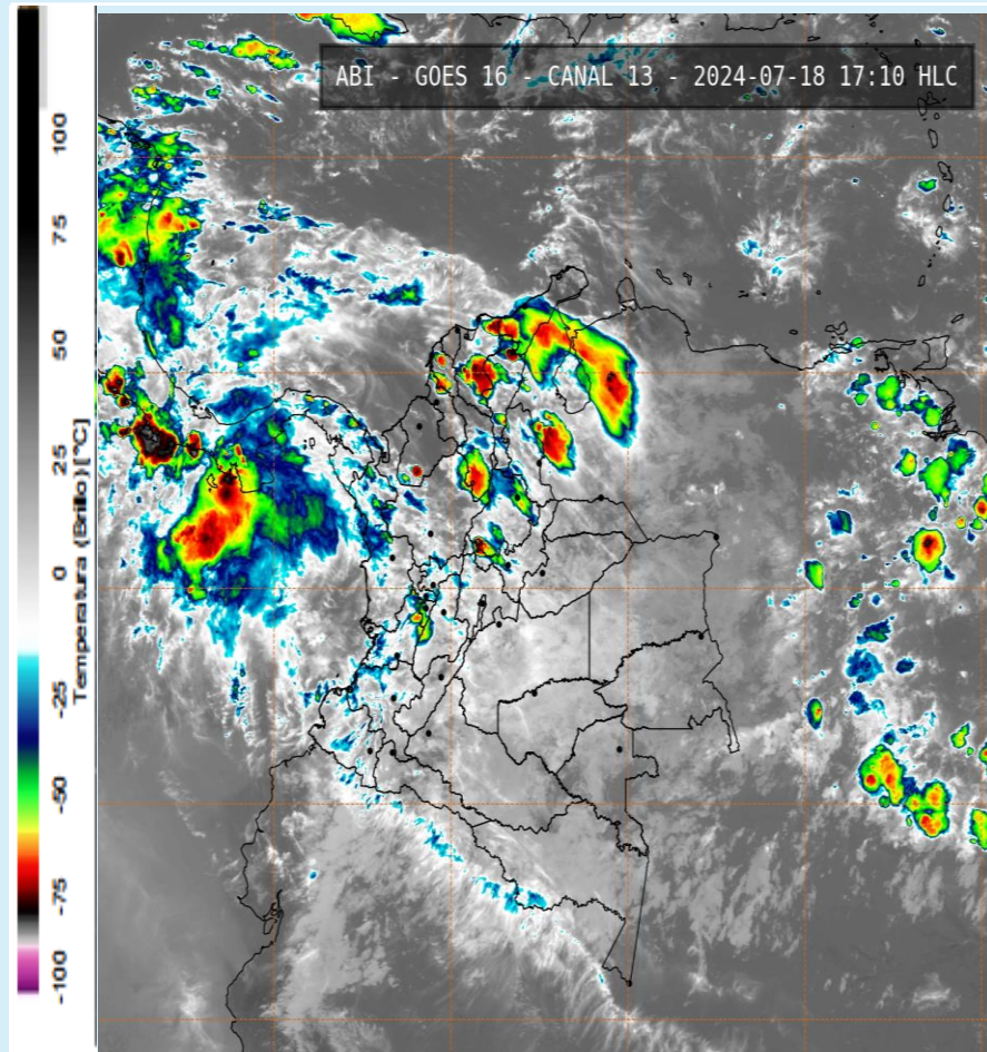
Imagen GOES 16 (East) Canal Infrarrojo | Fuente: GOES-IDEAM 18 de julio de 2024- Hora 17:10 HLC
