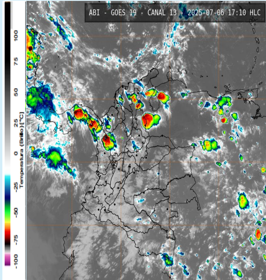
Imagen GOES 19 (East) Canal Infrarrojo 6 de julio de 2025 - Hora 17:10 HLC Fuente: IDEAM
