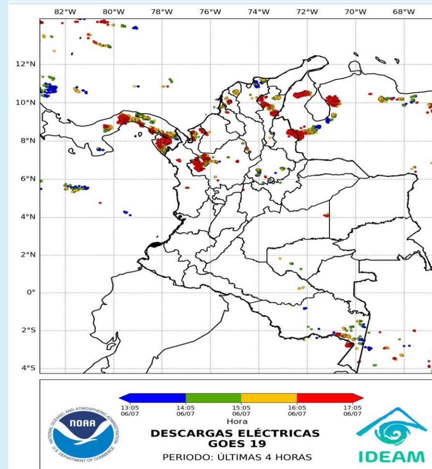
Descargas eléctricas 6 de julio de 2025 - Hora 17:30 HLC Fuente: IDEAM
