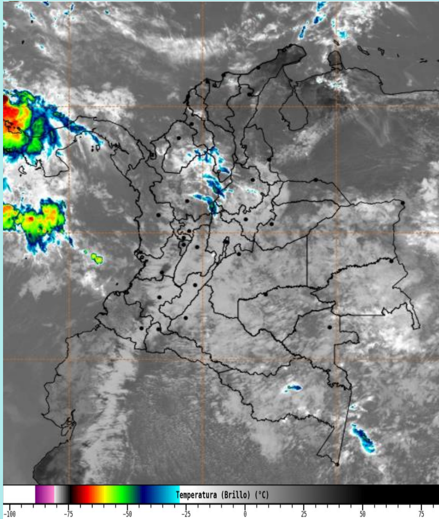
Imagen GOES East Canal Infrarrojo, 6 de julio de 2025 - Hora 12:00 HLC. Fuente: IDEAM - GOES 19
