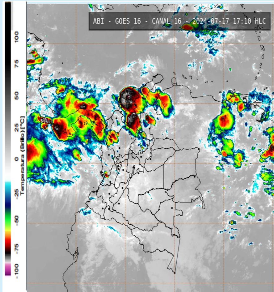
Imagen GOES 16 (East) Canal Infrarrojo | Fuente: GOES-IDEAM 17 de julio de 2024- Hora 17:10 HLC
