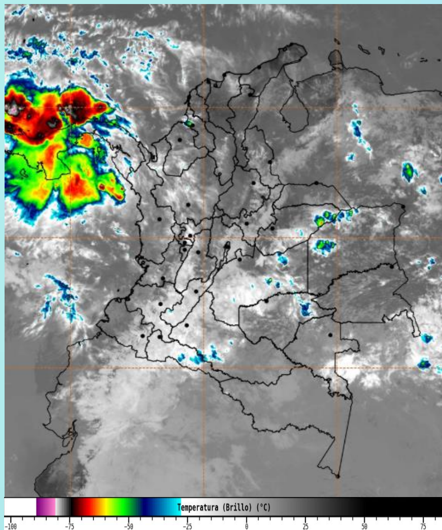
Imagen GOES East Canal Infrarrojo, 2 de julio de 2025 - Hora 11:40 HLC. Fuente: IDEAM - GOES 19
