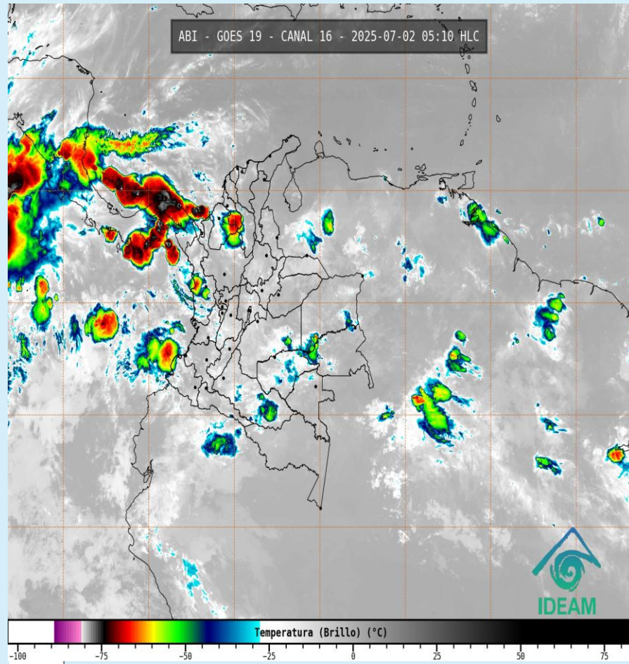
Imagen GOES 19 (East) Canal Infrarrojo 2 de julio de 2025 - Hora 05:20 HLC Fuente: IDEAM
