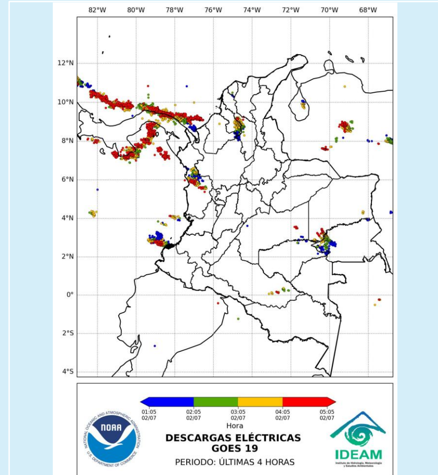
Descargas eléctricas 2 de julio de 2025 – Hora 05:10 HLC Fuente: IDEAM
