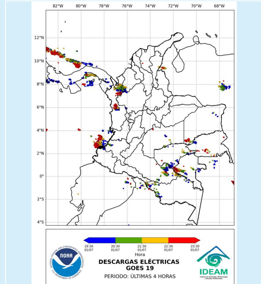
Descargas eléctricas 1 de julio de 2025 - Hora 23:30 HLC Fuente: IDEAM
