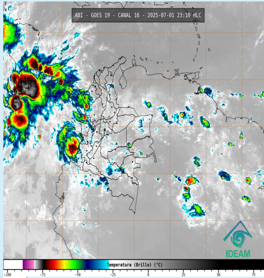
Imagen GOES 19 (East) Canal Infrarrojo 1 de julio de 2025 - Hora 23:10 HLC Fuente: IDEAM
