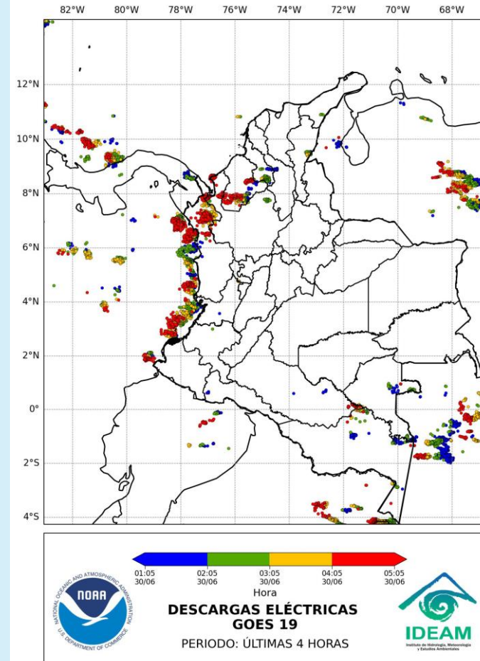
Descargas eléctricas 30 de junio de 2025 – Hora 05:10 HLC Fuente: IDEAM
