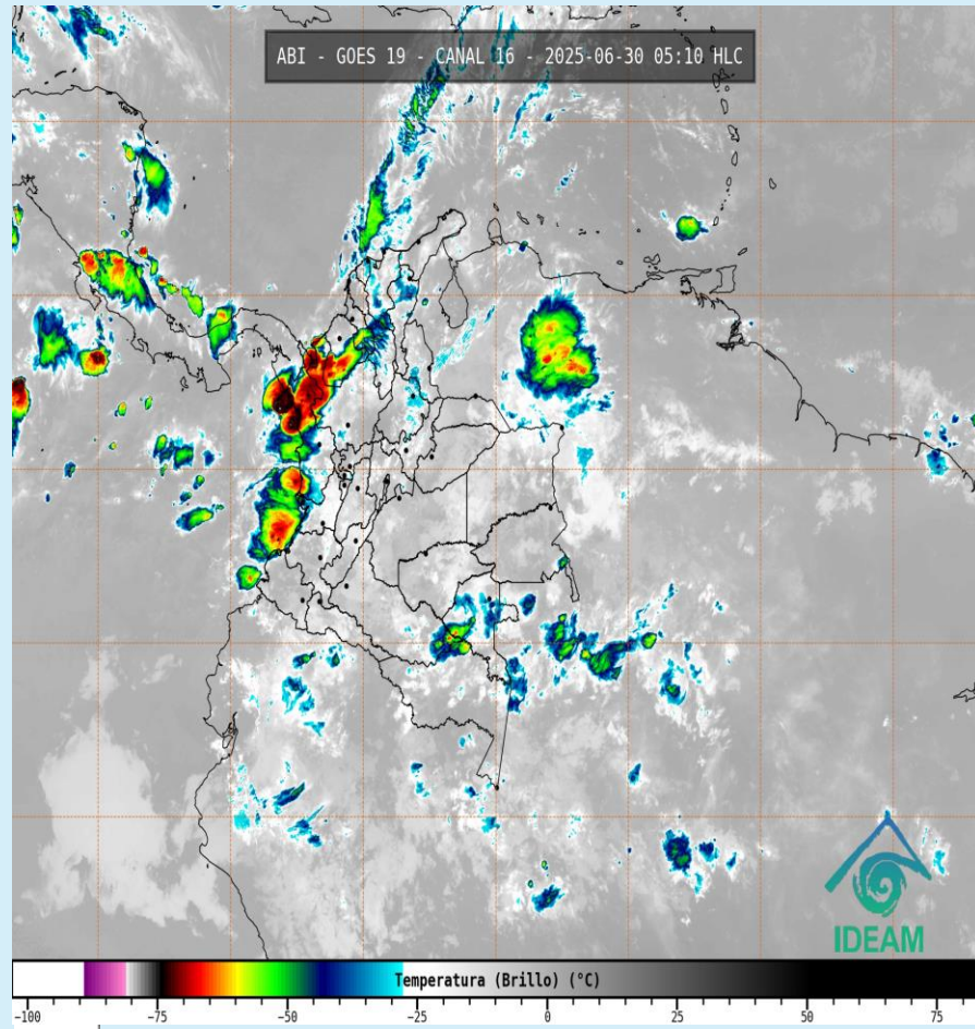
Imagen GOES 19 (East) Canal Infrarrojo 30 de junio de 2025 - Hora 05:10 HLC Fuente: IDEAM
