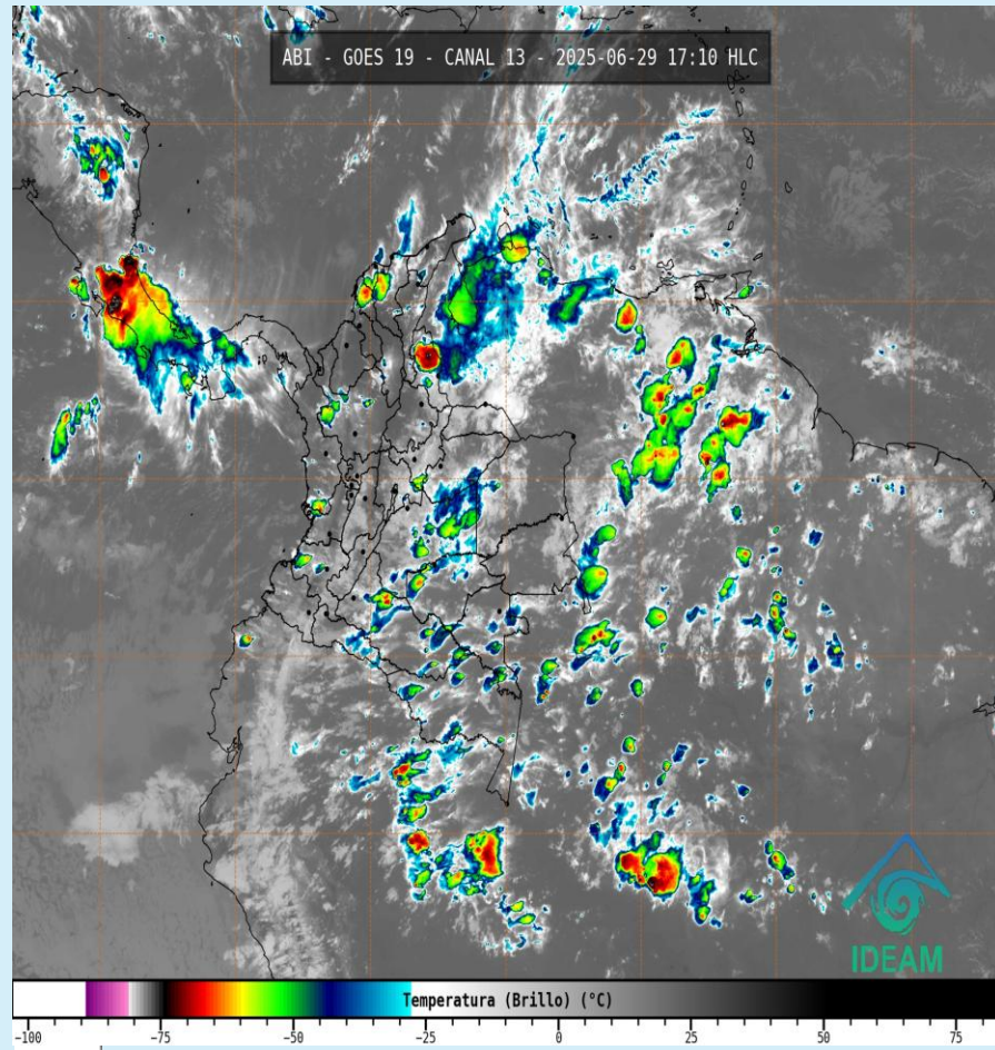
Imagen GOES 19 (East) Canal Infrarrojo 29 de junio de 2025 - Hora 17:10 HLC Fuente: IDEAM
