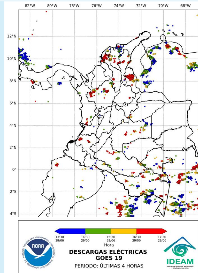
Descargas eléctricas 29 de junio de 2025 – Hora 17:45 HLC Fuente: IDEAM
