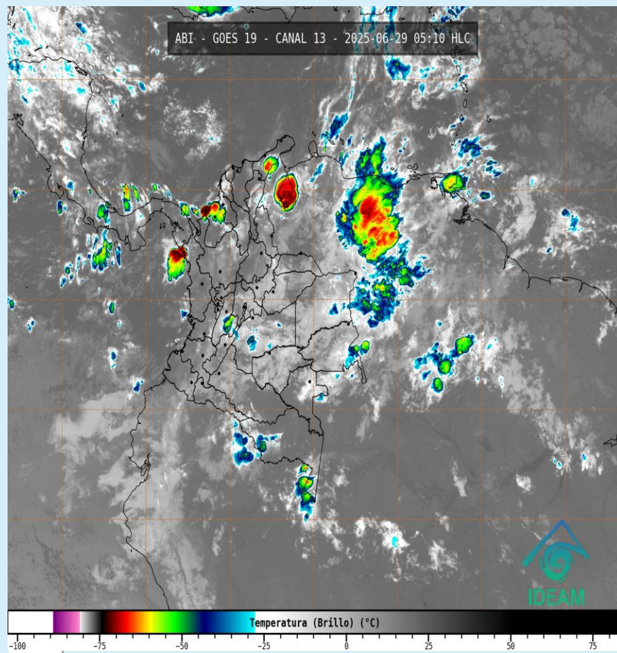
Imagen GOES 19 (East) Canal Infrarrojo 29 de junio de 2025 - Hora 05:10 HLC Fuente: IDEAM
