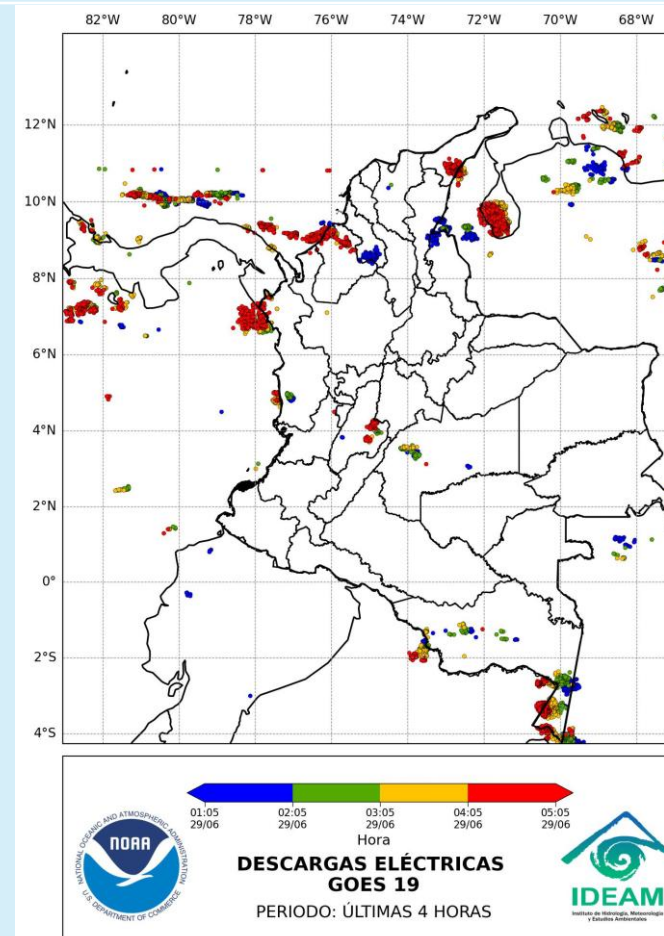
Descargas eléctricas 29 de junio de 2025 – Hora 05:05 HLC Fuente: IDEAM
