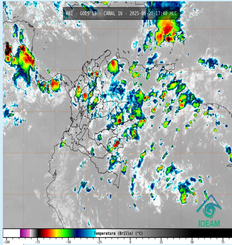
Imagen GOES 19 (East) Canal Infrarrojo 28 de junio de 2025 - Hora 17:40 HLC Fuente: IDEAM
