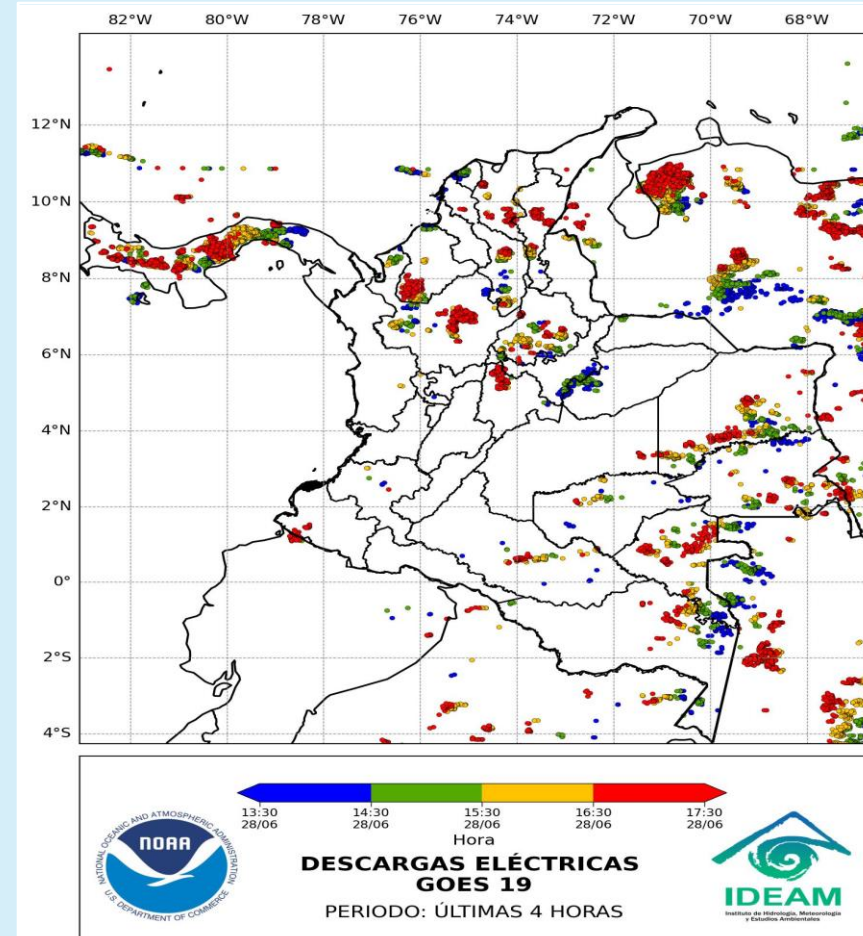
Descargas eléctricas 28 de junio de 2025 – Hora 17:30 HLC Fuente: IDEAM
