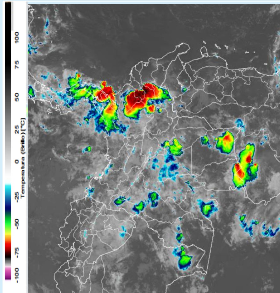
Imagen GOES 19 (East) Canal Infrarrojo 27 de junio de 2025 - Hora 23:20 HLC Fuente: https://rammb-slider.cira.colostate.edu/
