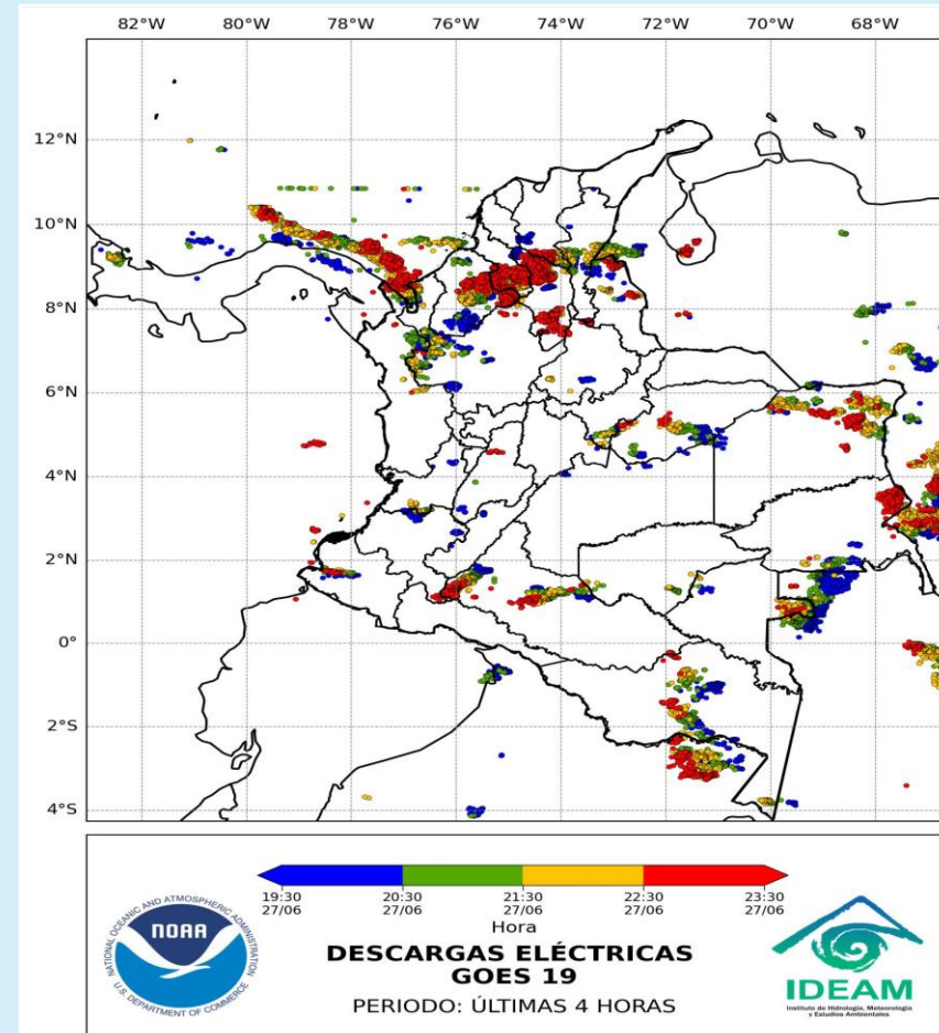
Descargas eléctricas 27 de junio de 2025 – Hora 23:37 HLC Fuente: IDEAM
