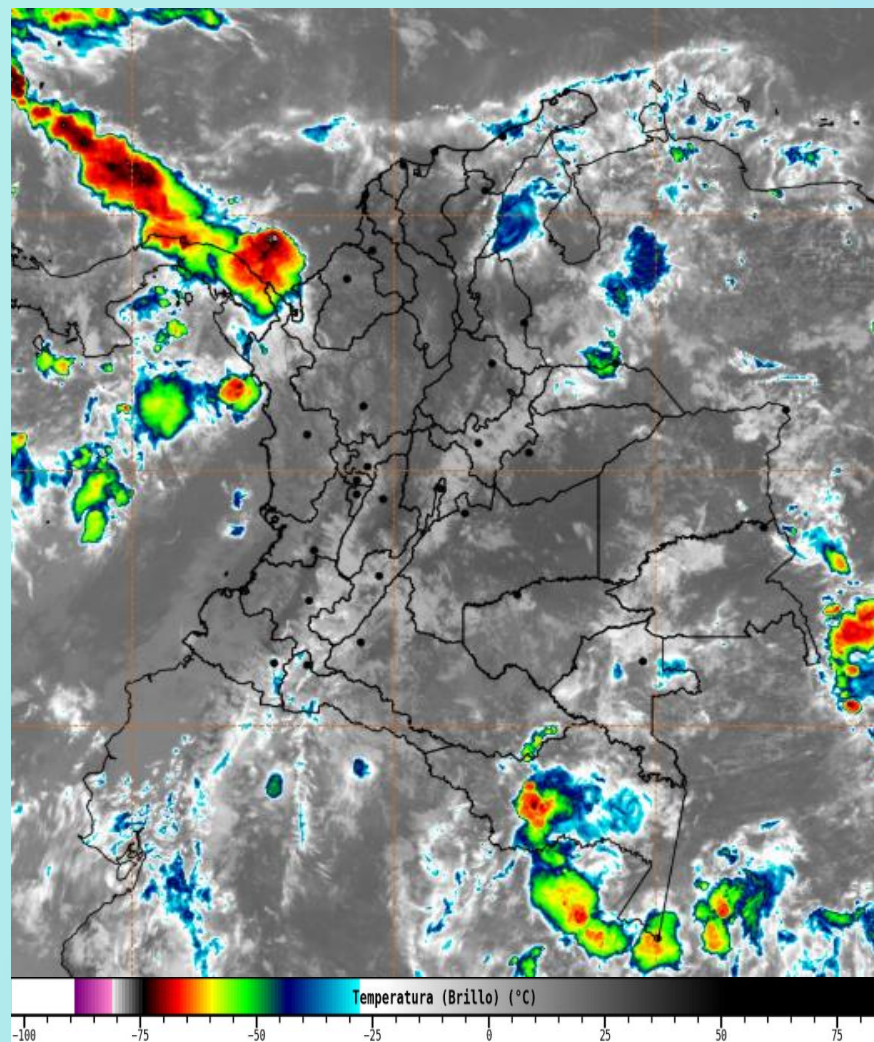
Imagen GOES East Canal Infrarrojo, 25 de junio de 2025 - Hora 11:20 HLC. Fuente: IDEAM - GOES 19
