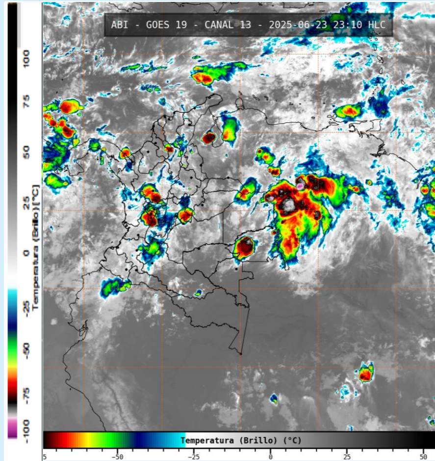
Imagen GOES 19 (East) Canal Infrarrojo 23 de junio de 2025 - Hora 23:10 HLC Fuente: IDEAM
