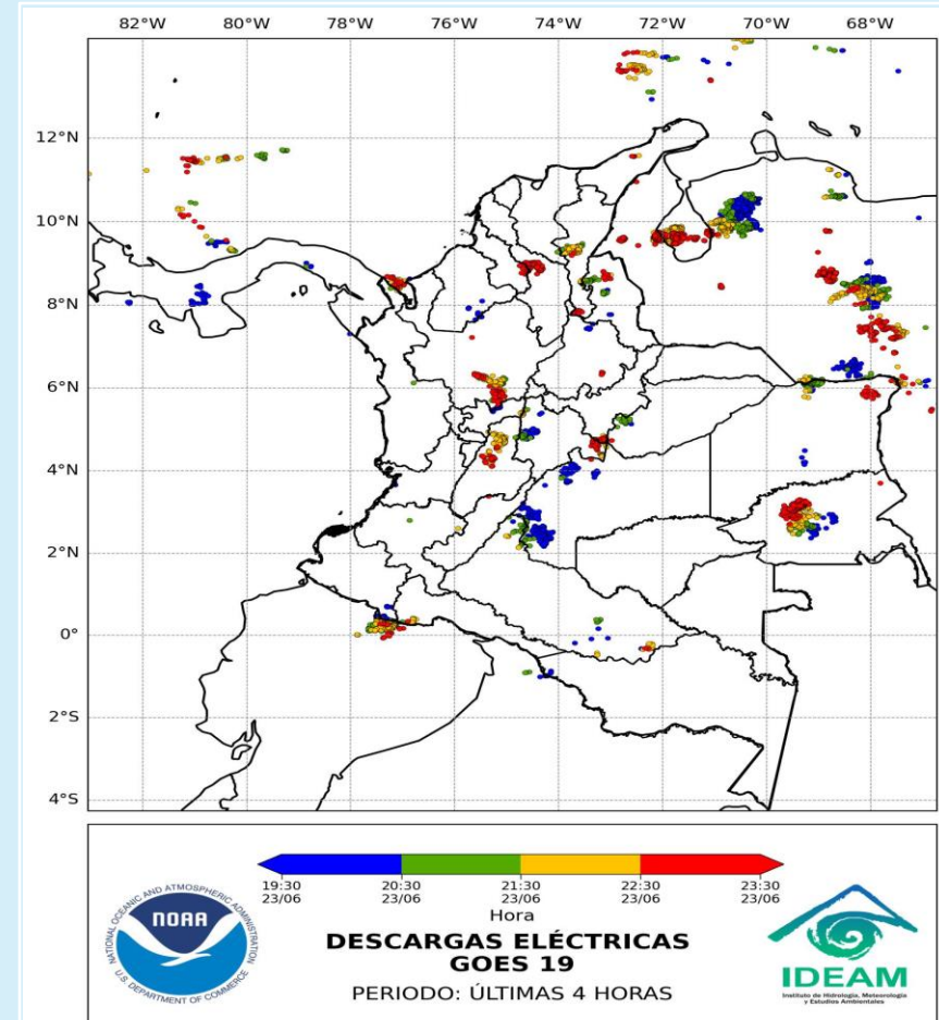
Descargas eléctricas 23 de junio de 2025 – Hora 22:05 HLC Fuente: IDEAM
