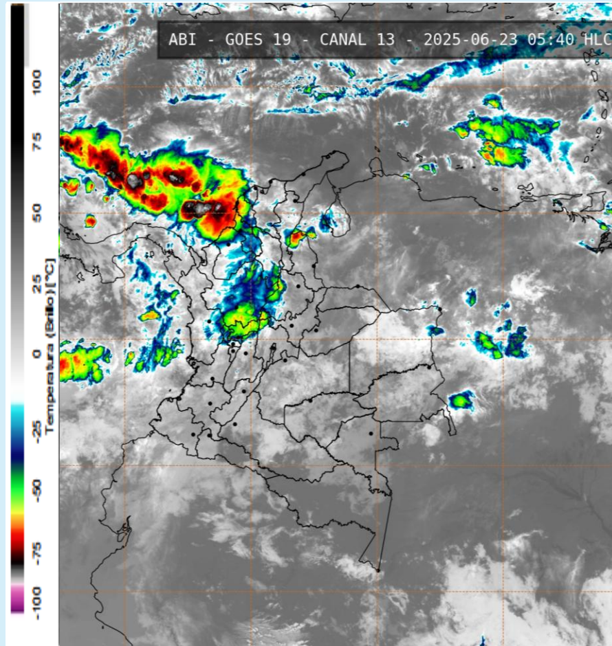
Imagen GOES 19 (East) Canal Infrarrojo 23 de junio de 2025 - Hora 05:40 HLC Fuente: IDEAM
