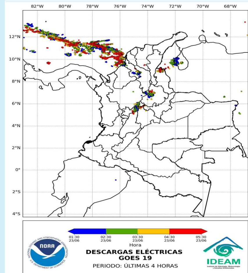
Descargas eléctricas 23 de junio de 2025 – Hora 05:30 HLC Fuente: IDEAM
