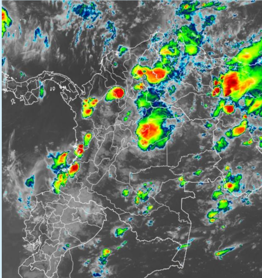
Imagen GOES 19 (East) Canal Infrarrojo 19 de junio de 2025- Hora 17:30 HLC Fuente: CIRA
