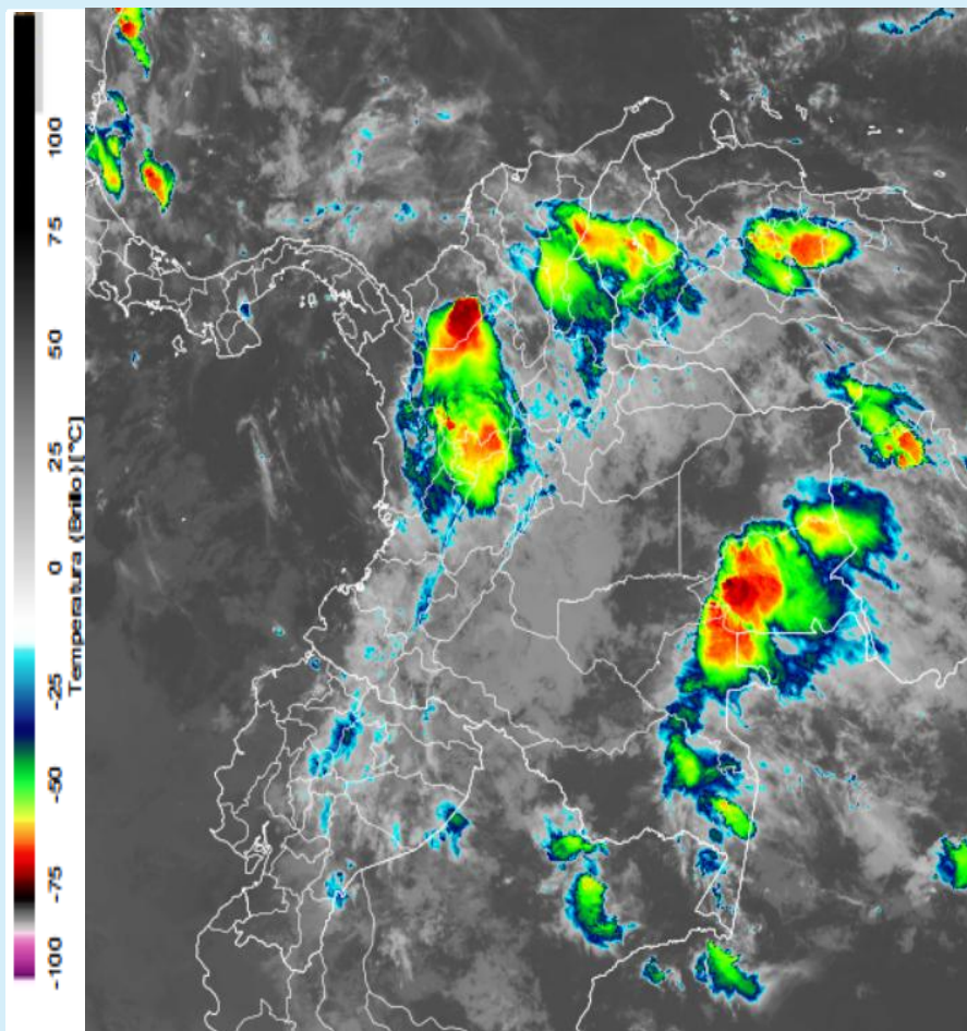
Imagen GOES 19 (East) Canal Infrarrojo 17 de junio de 2025- Hora 23:10 HLC Fuente: IDEAM
