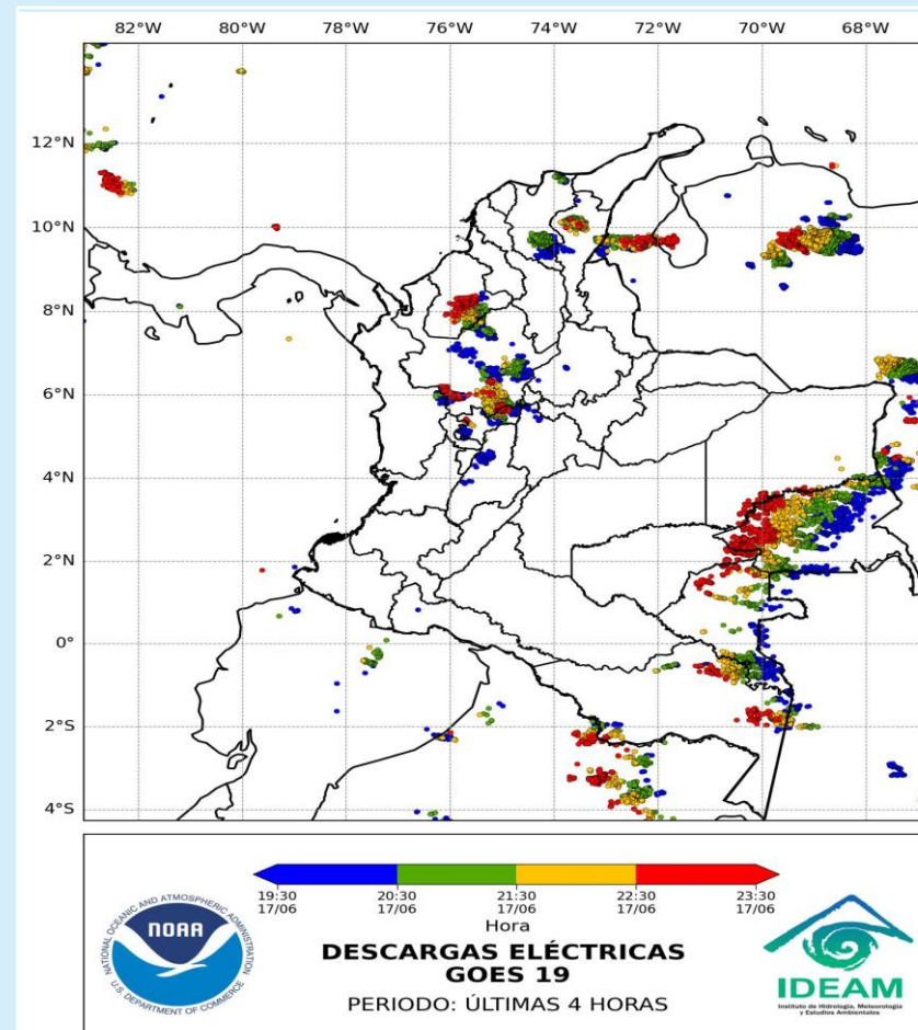
Descargas eléctricas 17 de junio de 2025- Hora 23:05 HLC Fuente: IDEAM
