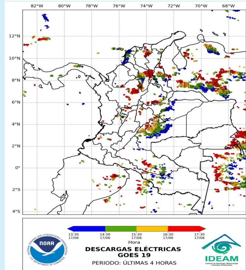
Descargas eléctricas 17 de junio de 2025- Hora 17:30 HLC Fuente: IDEAM
