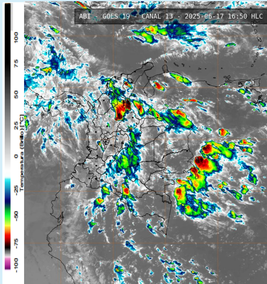
Imagen GOES 19 (East) Canal Infrarrojo 17 de junio de 2025- Hora 16:50 HLC Fuente: IDEAM
