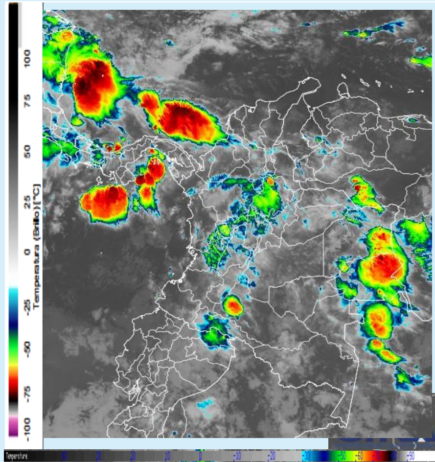
Imagen GOES 19 (East) Canal Infrarrojo 17 de junio de 2025- Hora 05:25 HLC Fuente: rammb-slider.cira.colostate.edu
