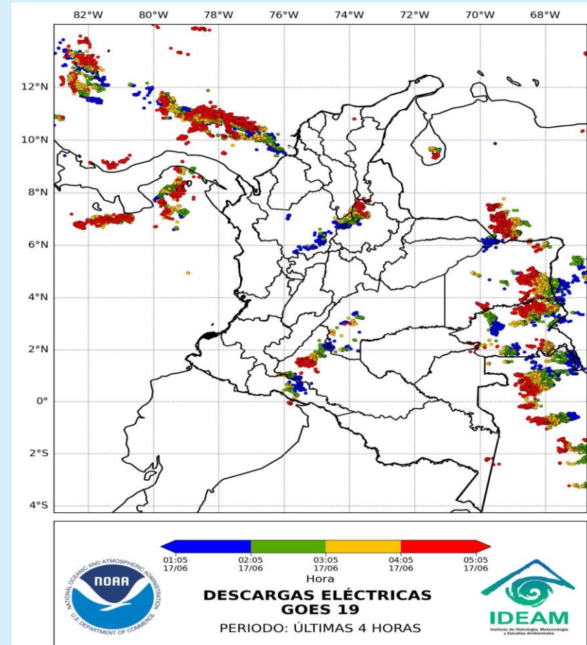
Descargas eléctricas 17 de junio de 2025- Hora 05:30 HLC Fuente: IDEAM
