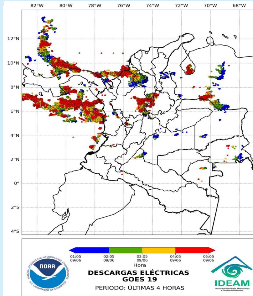
Descargas eléctricas 9 de junio de 2025- Hora 05:30 HLC Fuente: IDEAM
