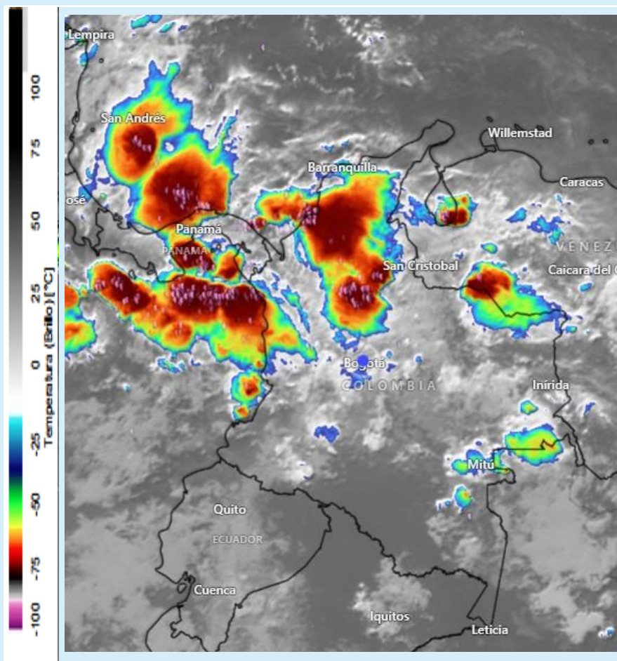
Imagen GOES 19 (East) Canal Infrarrojo 9 de junio de 2025- Hora 05:40 HLC Fuente: WINDY
