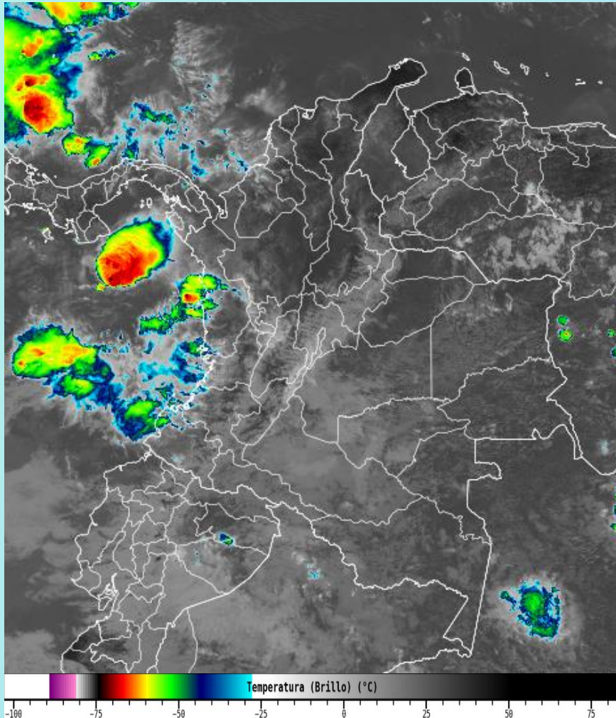
Imagen GOES East Canal Infrarrojo, 8 de junio de 2025 - Hora 11:50 HLC. Fuente: IDEAM GOES 19
