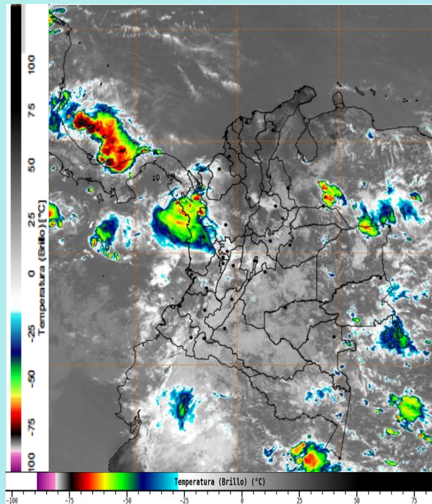
Imagen GOES East Canal Infrarrojo, 23 de mayo de 2025 - Hora 11:50 HLC. Fuente: IDEAM GOES -19
