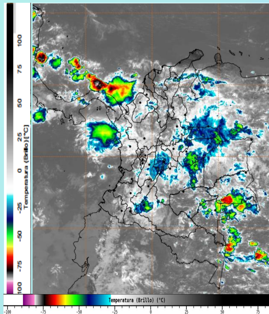
Imagen GOES East Canal Infrarrojo, 22 de mayo de 2025 - Hora 11:10 HLC. Fuente: IDEAM GOES -19
