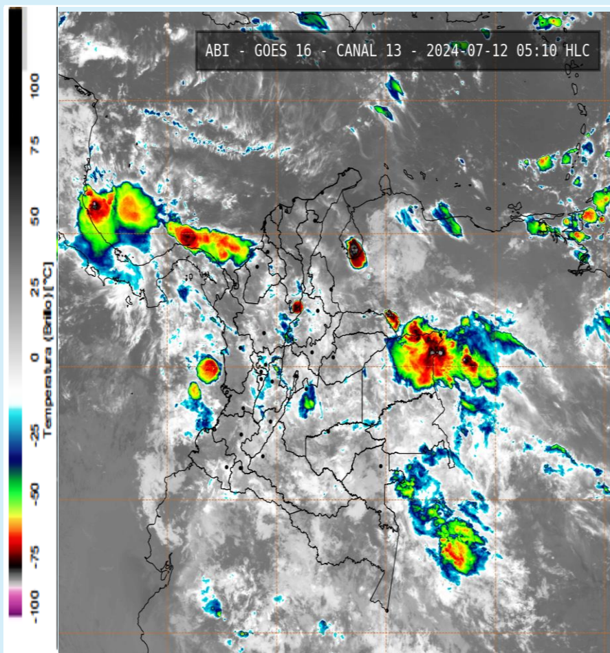
Imagen GOES 16 (East) Canal Infrarrojo | Fuente: GOES-IDEAM 12 de julio de 2024- Hora 05:10 HLC
