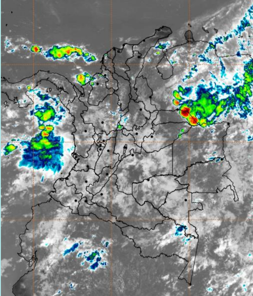
Imagen GOES East Canal Infrarrojo, 18 de mayo de 2025 - Hora 11:40 HLC. Fuente: IDEAM GOES -19
