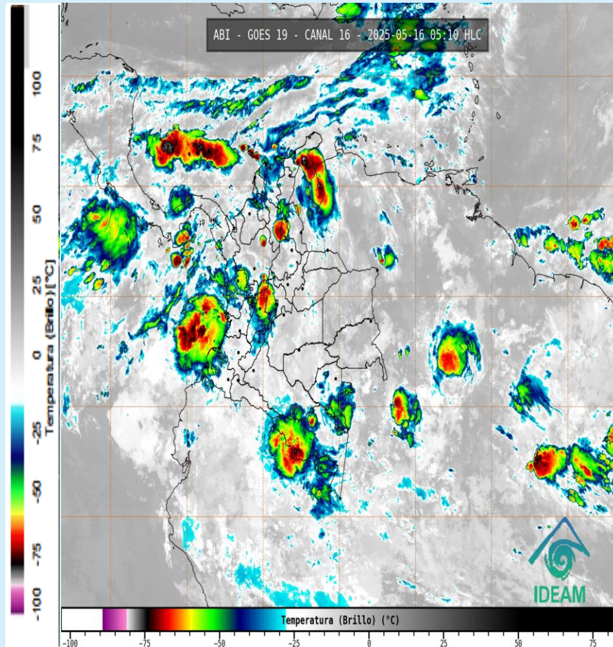
Imagen GOES 19 (East) Canal Infrarrojo 16 de mayo de 2025 - Hora 05:10 HLC Fuente: IDEAM GOES-19
