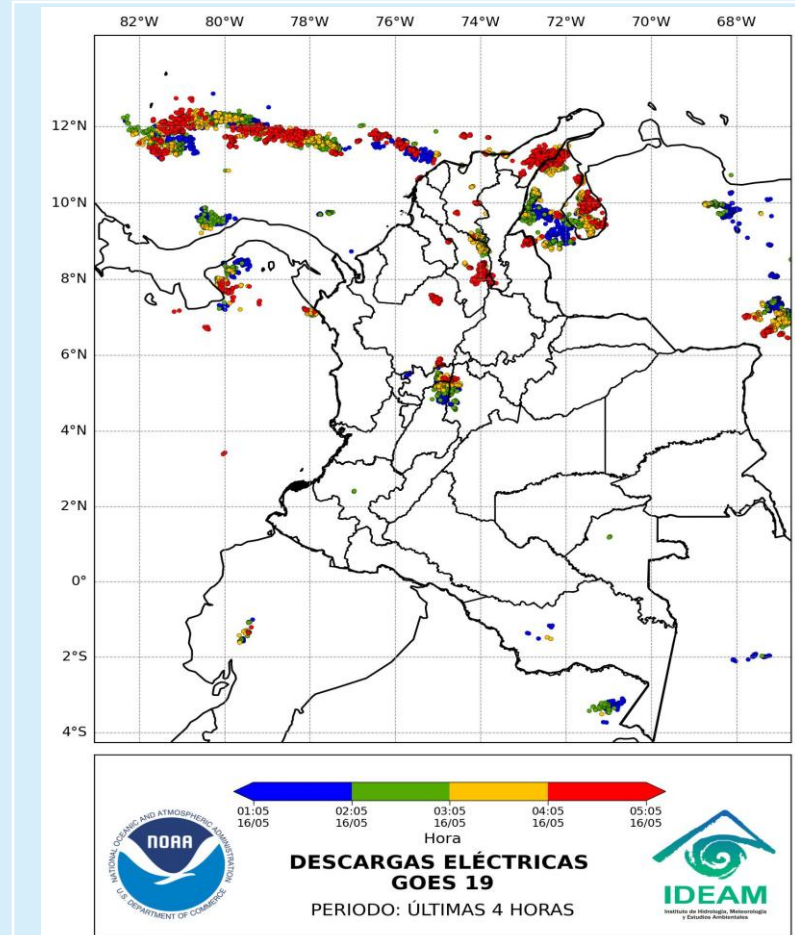
Descargas eléctricas 16 de mayo de 2025 - Hora 05:03 HLC Fuente: IDEAM
