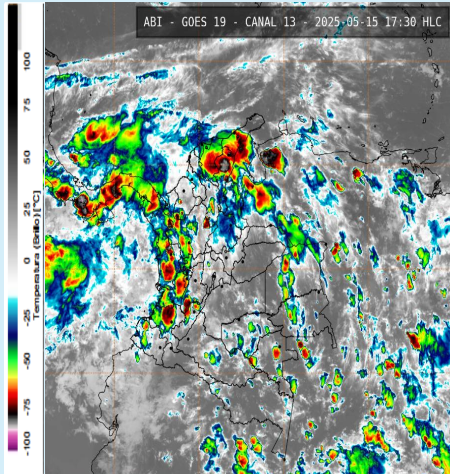
Imagen GOES 19 (East) Canal Infrarrojo 15 de mayo de 2025 - Hora 17:30 HLC Fuente: IDEAM GOES-19
