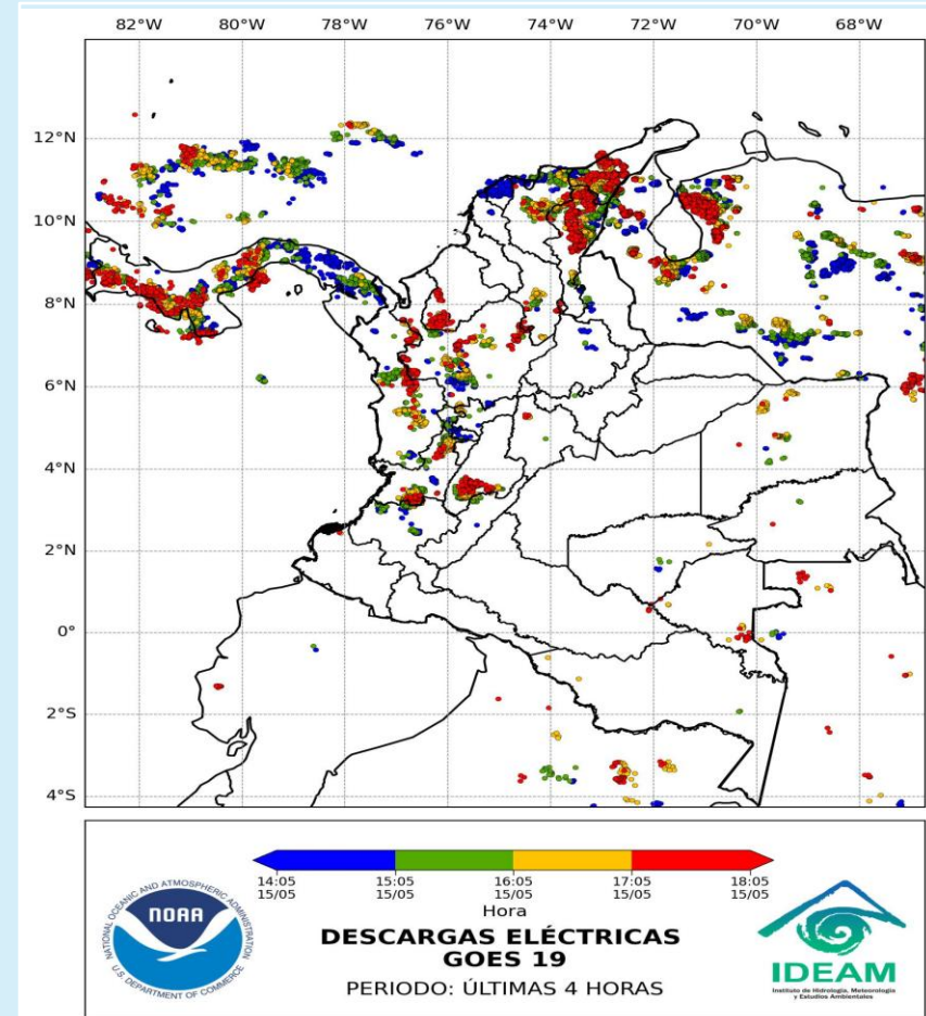
Descargas eléctricas 15 de mayo de 2025 – Hora 05:30 HLC Fuente: IDEAM
