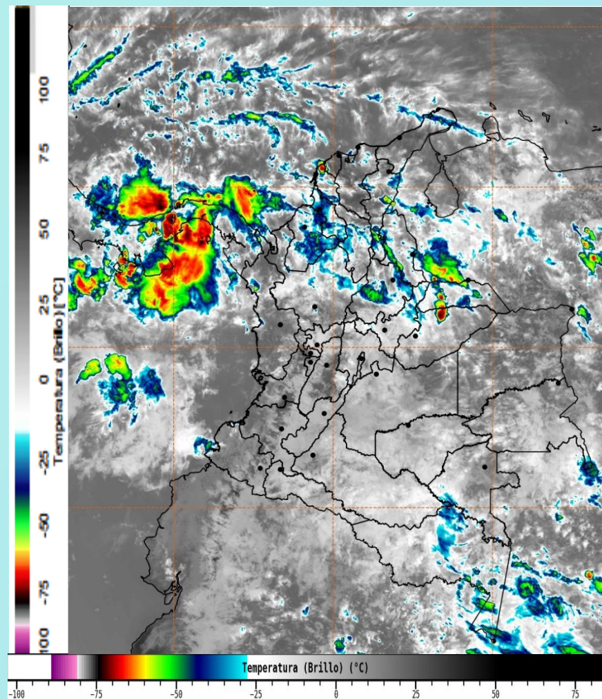
Imagen GOES East Canal Infrarrojo, 14 de mayo de 2025 - Hora 12:10 HLC. Fuente: IDEAM GOES -19
