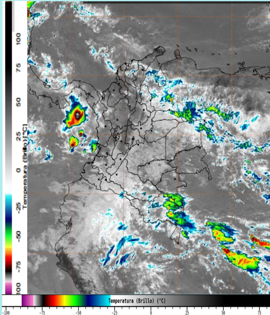
Imagen GOES East Canal Infrarrojo, 12 de mayo de 2025 - Hora 11:30 HLC. Fuente: IDEAM GOES -19
