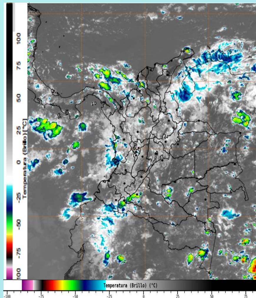
Imagen GOES East Canal Infrarrojo, 8 de mayo de 2025 - Hora 12:00 HLC. Fuente: IDEAM GOES -19
