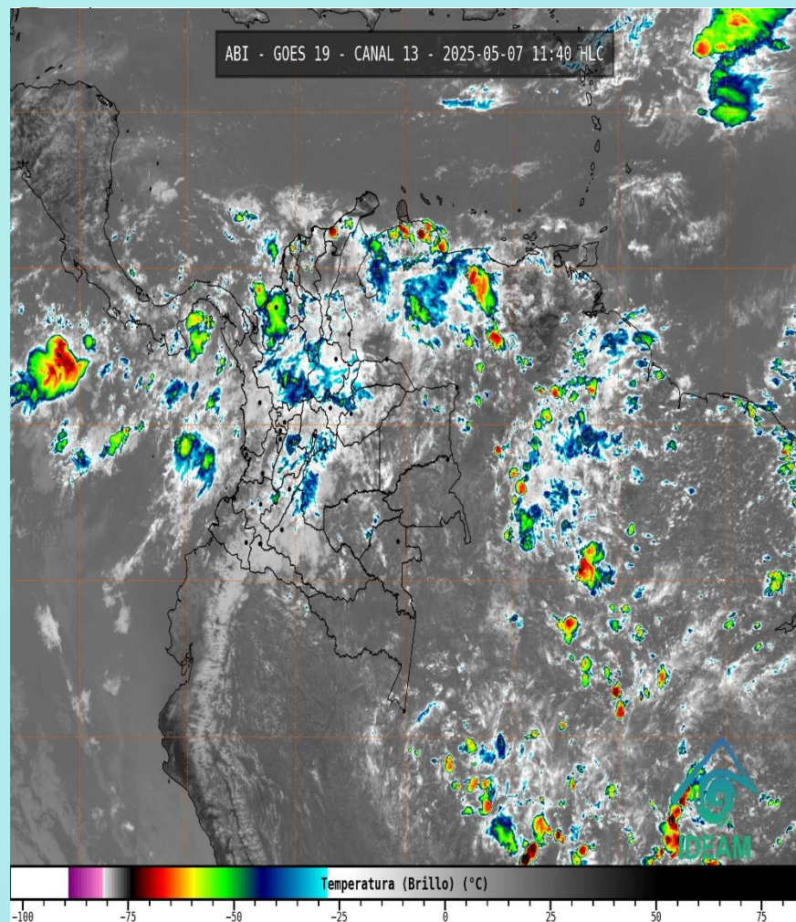
Imagen GOES East Canal Infrarrojo, 7 de mayo de 2025 - Hora 11:40 HLC. Fuente: IDEAM GOES -19
