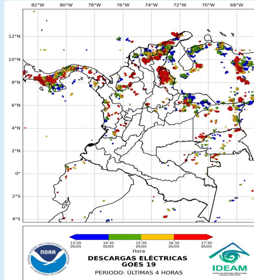
Descargas eléctricas 04 mayo de 2025 – Hora 17:30 HLC Fuente: IDEAM
