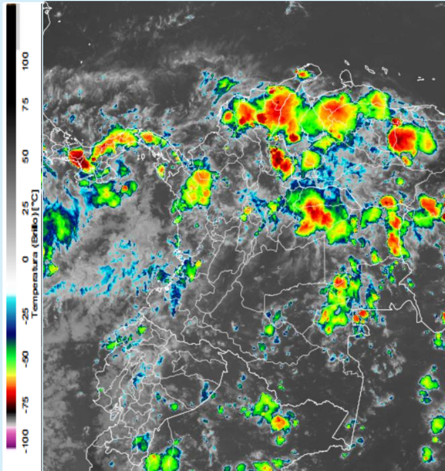
Imagen GOES 19 (East) Canal Infrarrojo 5 de mayo de 2025 - Hora 17:30 HLC Fuente: IDEAM GOES-19
