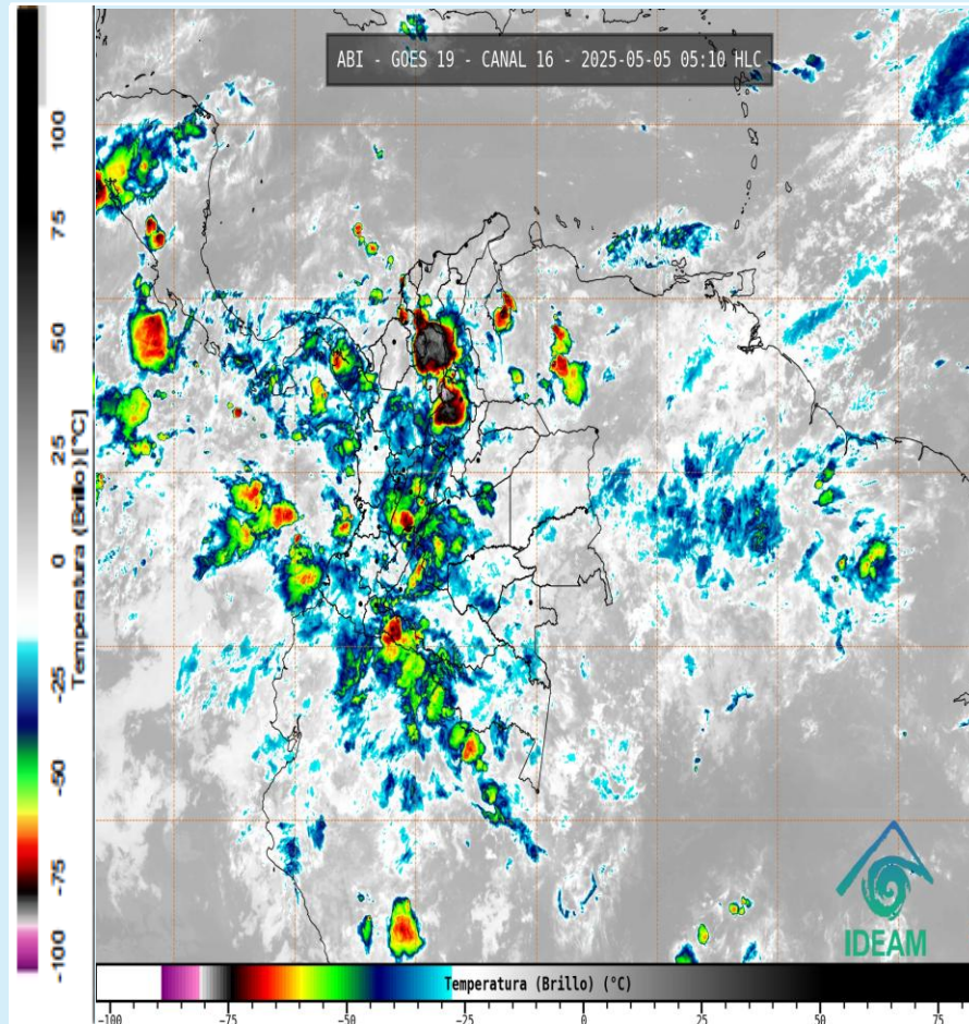
Imagen GOES 19 (East) Canal Infrarrojo 5 de mayo de 2025 - Hora 05:10 HLC Fuente: IDEAM GOES-19
