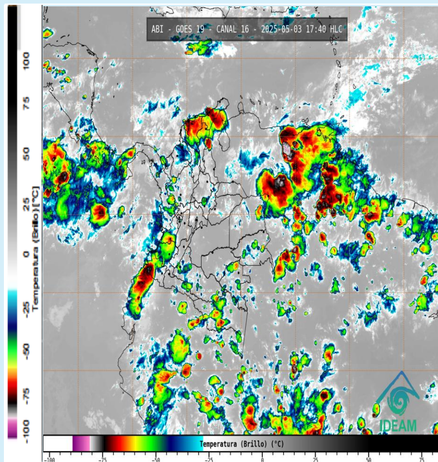
Imagen GOES 19 (East) Canal Infrarrojo 3 de mayo de 2025 - Hora 17:40 HLC Fuente: IDEAM GOES-19
