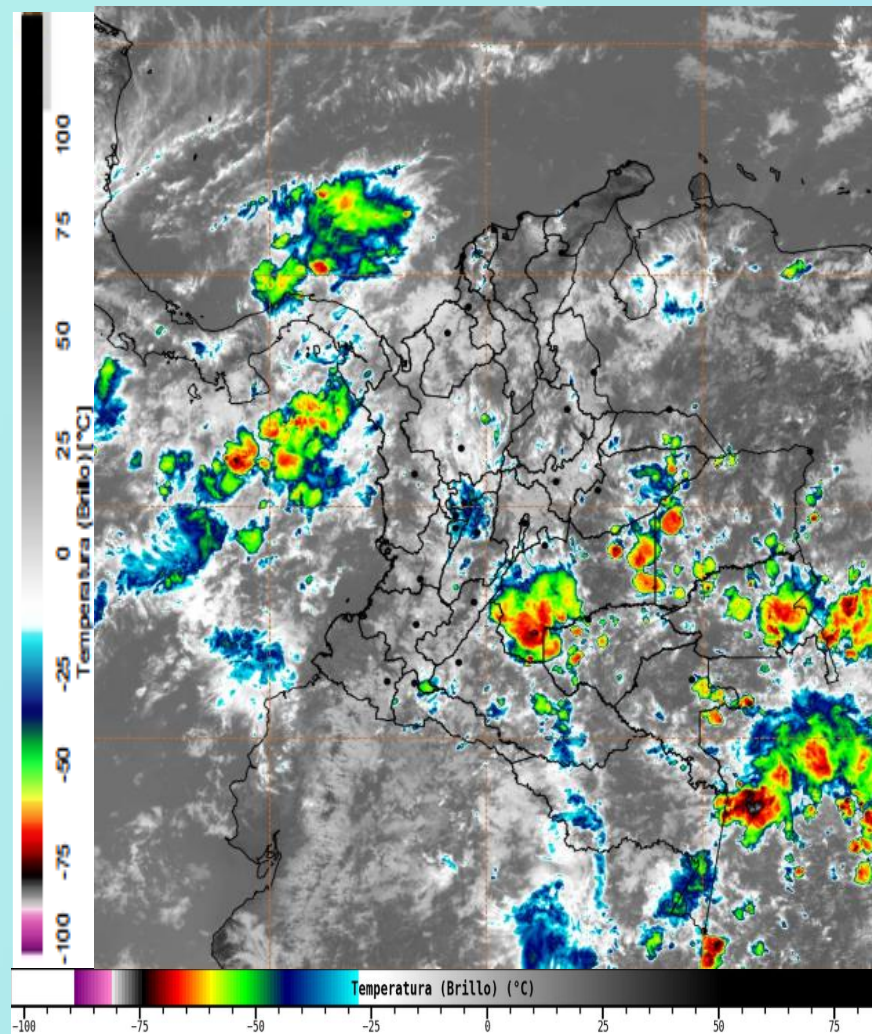
Imagen GOES East Canal Infrarrojo, 3 de mayo de 2025 - Hora 12:00 HLC. Fuente: IDEAM GOES -19
