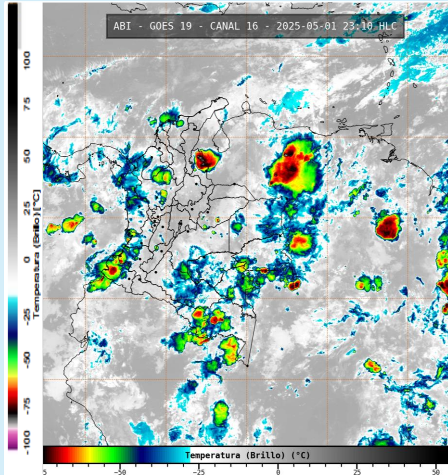
Imagen GOES 19 (East) Canal Infrarrojo 01 mayo de 2025 - Hora 23:10 HLC Fuente: IDEAM GOES-19
