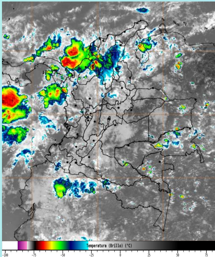
Imagen GOES East Canal Infrarrojo, 1 de mayo de 2025 - Hora 11:50 HLC. Fuente: IDEAM GOES -19
