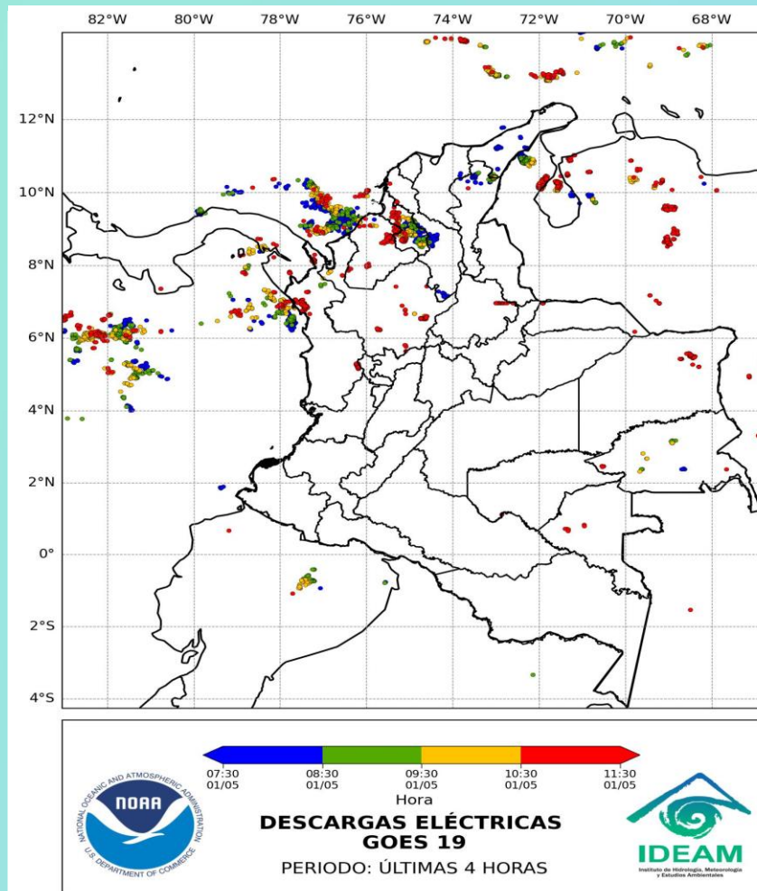
Descargas eléctricas en las últimas cuatro horas. Hora 11:30 HLC Fuente: IDEAM
