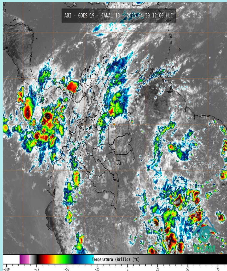
Imagen GOES East Canal Infrarrojo, 30 de abril de 2025 - Hora 12:00 HLC. Fuente: IDEAM GOES -19
