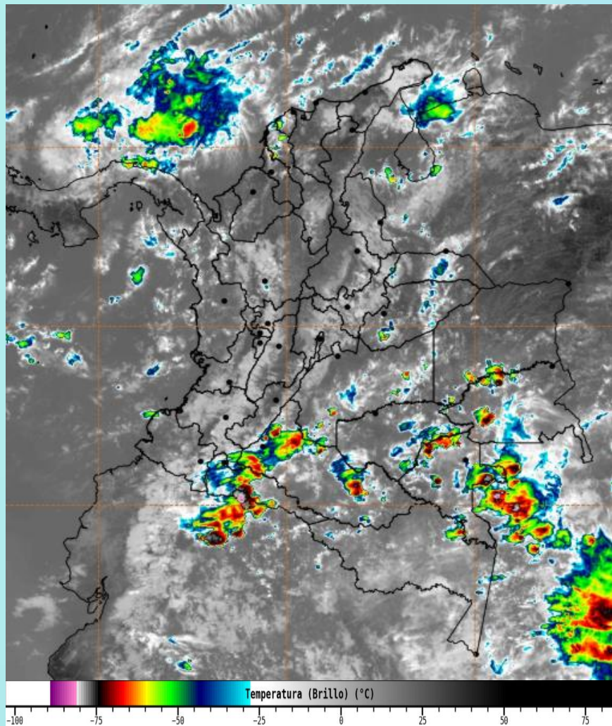
Imagen GOES East Canal Infrarrojo, 27 de abril de 2025 - Hora 12:00 HLC. Fuente: IDEAM GOES -19
