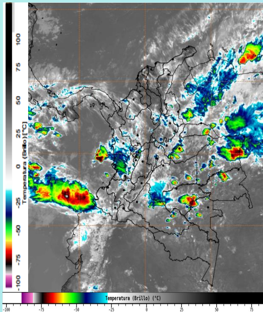
Imagen GOES East Canal Infrarrojo, 25 de abril de 2025 - Hora 11:50 HLC. Fuente: IDEAM GOES -19
