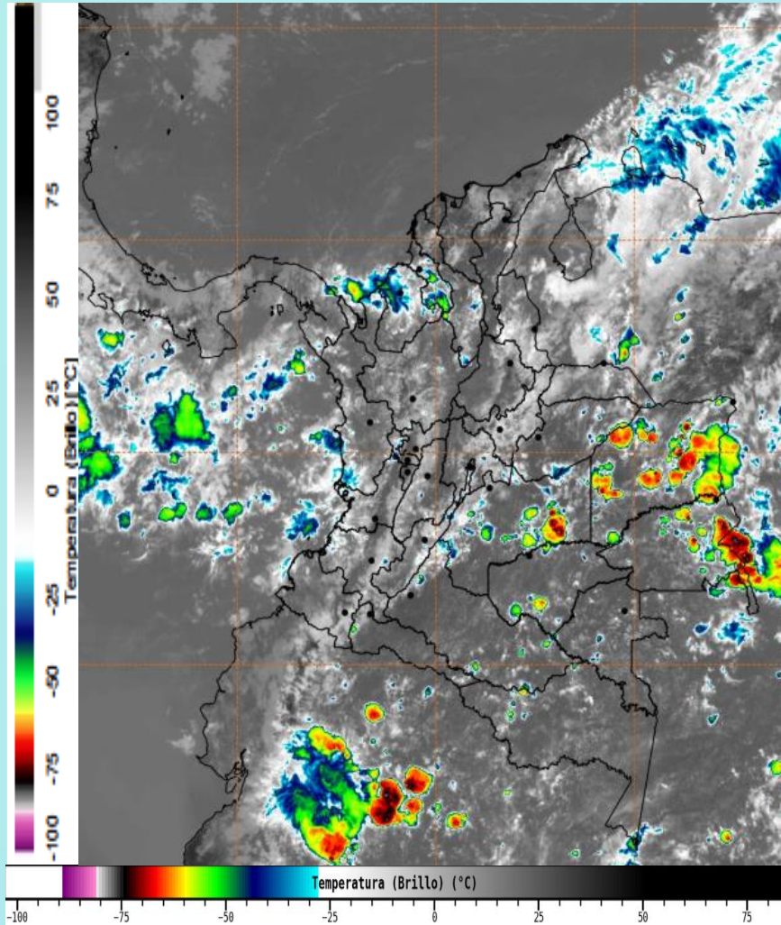
Imagen GOES East Canal Infrarrojo, 23 de abril de 2025 - Hora 11:50 HLC. Fuente: IDEAM GOES -19
