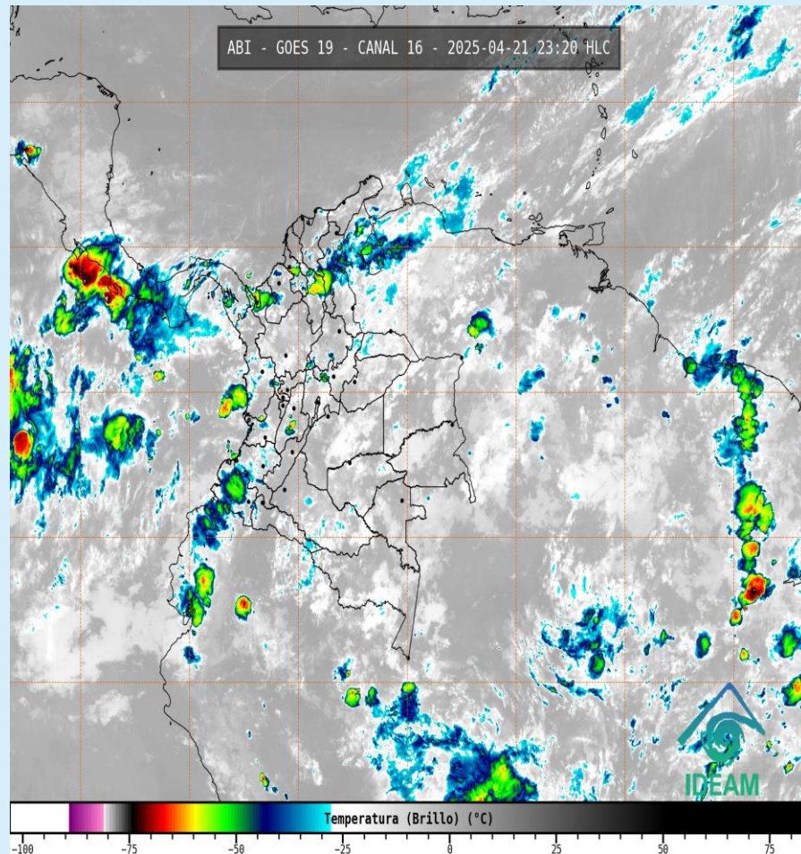
Imagen GOES 19 (East) Canal Infrarrojo 21 de abril de 2025 - Hora 23:20 HLC Fuente: IDEAM GOES-19
