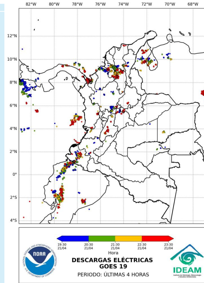
Descargas eléctricas 21 de abril de 2025 – 23:30 HLC Fuente: IDEAM
