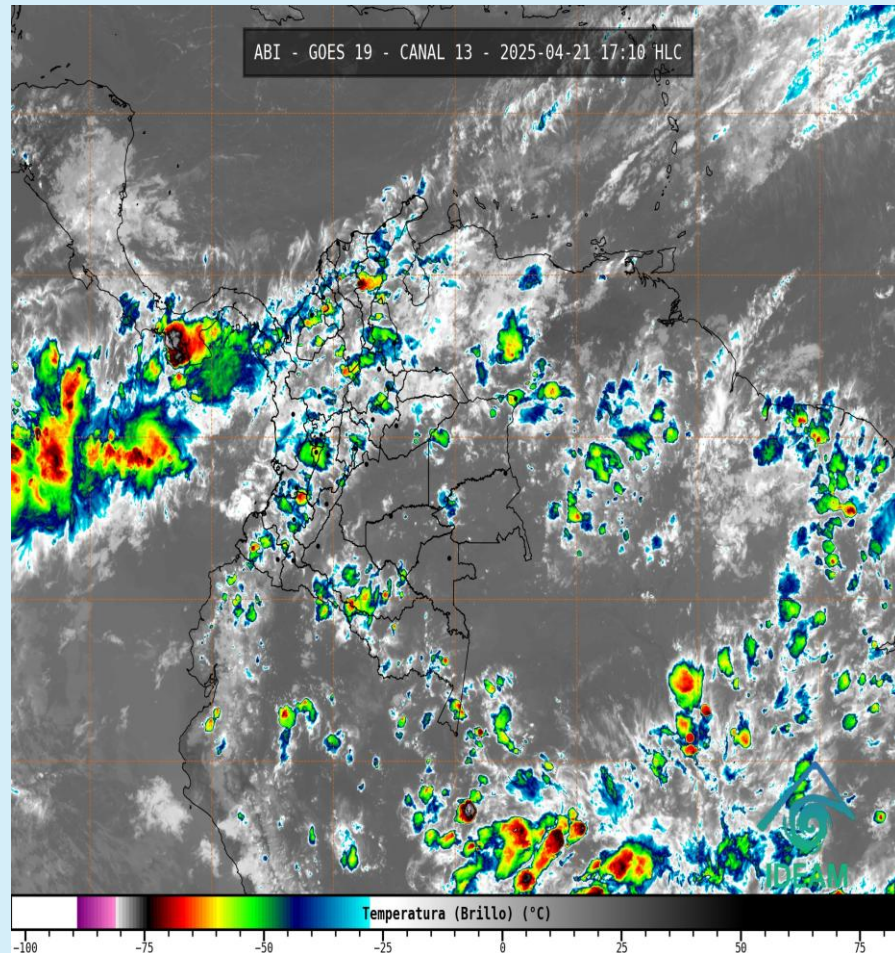
Imagen GOES 19 (East) Canal Infrarrojo 21 de abril de 2025 - Hora 17:10 HLC Fuente: IDEAM GOES-19
