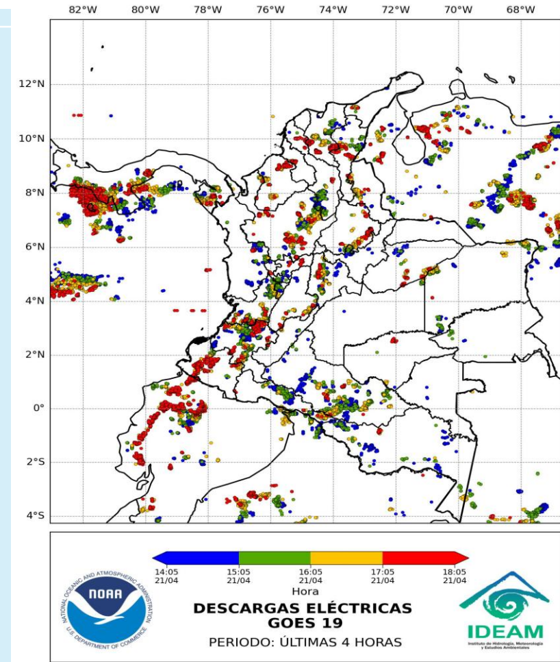
Descargas eléctricas 21 de abril de 2025 - 18:05 HLC Fuente: IDEAM
