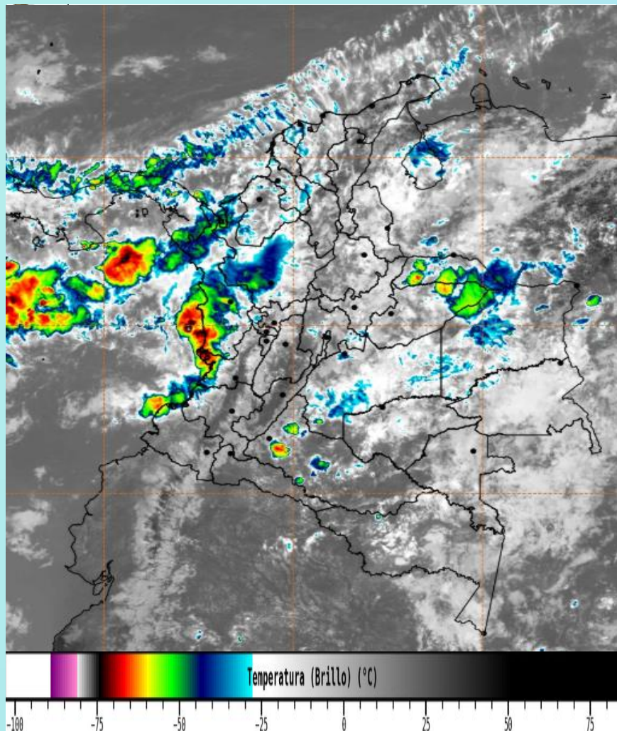
Imagen GOES East Canal Infrarrojo, 21 de abril de 2025 - Hora 11:40 HLC. Fuente: IDEAM GOES -19
