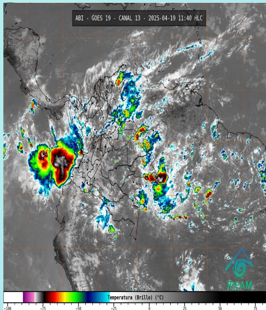
Imagen GOES East Canal Infrarrojo, 19 de abril de 2025 - Hora 11:40 HLC. Fuente: IDEAM GOES -19
