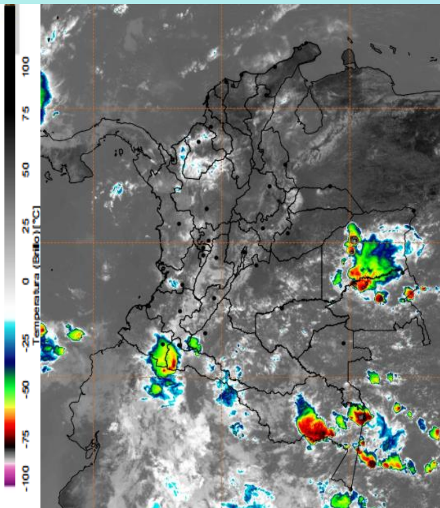
Imagen GOES East Canal Infrarrojo, 14 de abril de 2025 - Hora 11:35 HLC. Fuente: IDEAM GOES -19
