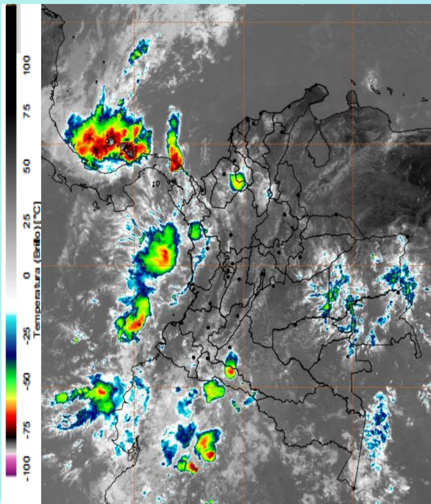
Imagen GOES East Canal Infrarrojo, 13 de abril de 2025 - Hora 11:50 HLC. Fuente: IDEAM GOES -19
