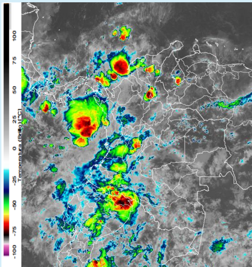
Imagen GOES 19 (East) Canal Infrarrojo 11 de abril de 2025 - Hora 05:00 HLC Fuente: Rammbslider
