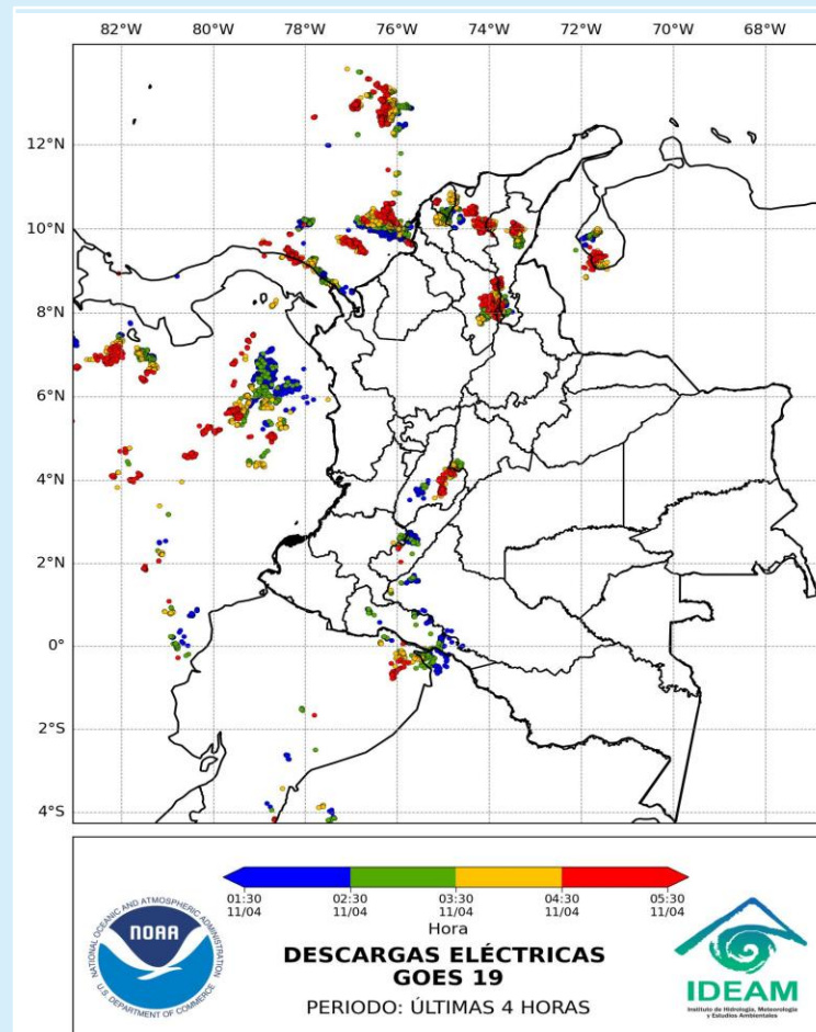
Descargas eléctricas últimas 4 horas 11 de abril de 2025 - Hora 05:30 HLC Fuente: IDEAM
